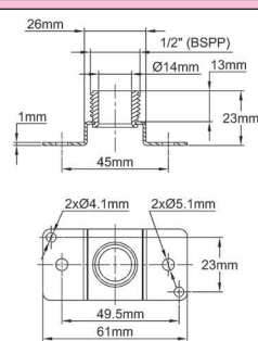
G \frac{1}{2} 圆棒散热器支架（用于空气管道安装）。 不使用在 Y0 的型号上。
