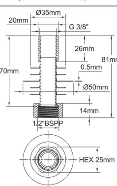
带 14.5 毫米端头的圆棒冷却器。 使用在高温的棒式温控器。适合安装在位于外壳下面的 \frac{3}{8} " 螺纹和直径 14.5 毫米的探温棒孔或法兰。 不使用在 Y0 的型号上。
