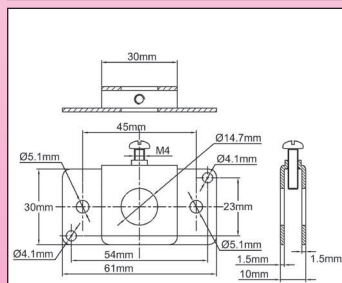
不锈钢法兰，用于直径 14.5 毫米的圆棒输出
