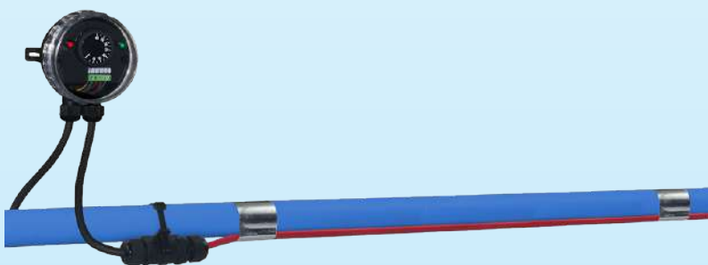
在一根伴热电缆的组装示例，带 Y24 接线盒，用于 PVC 管道的防冻保护
